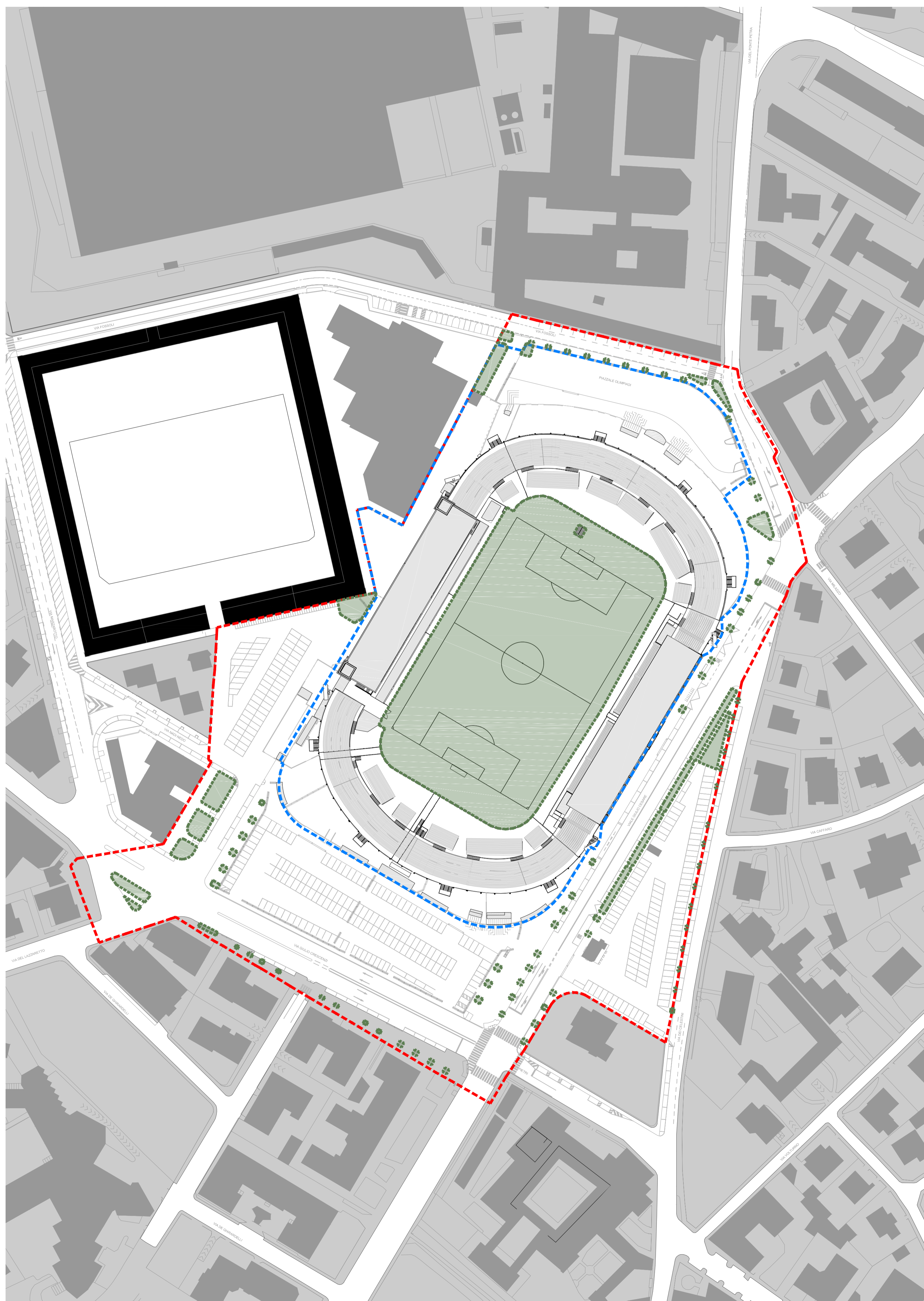
Planimetria di Stato di Fatto - Calcolo superficie drenante
