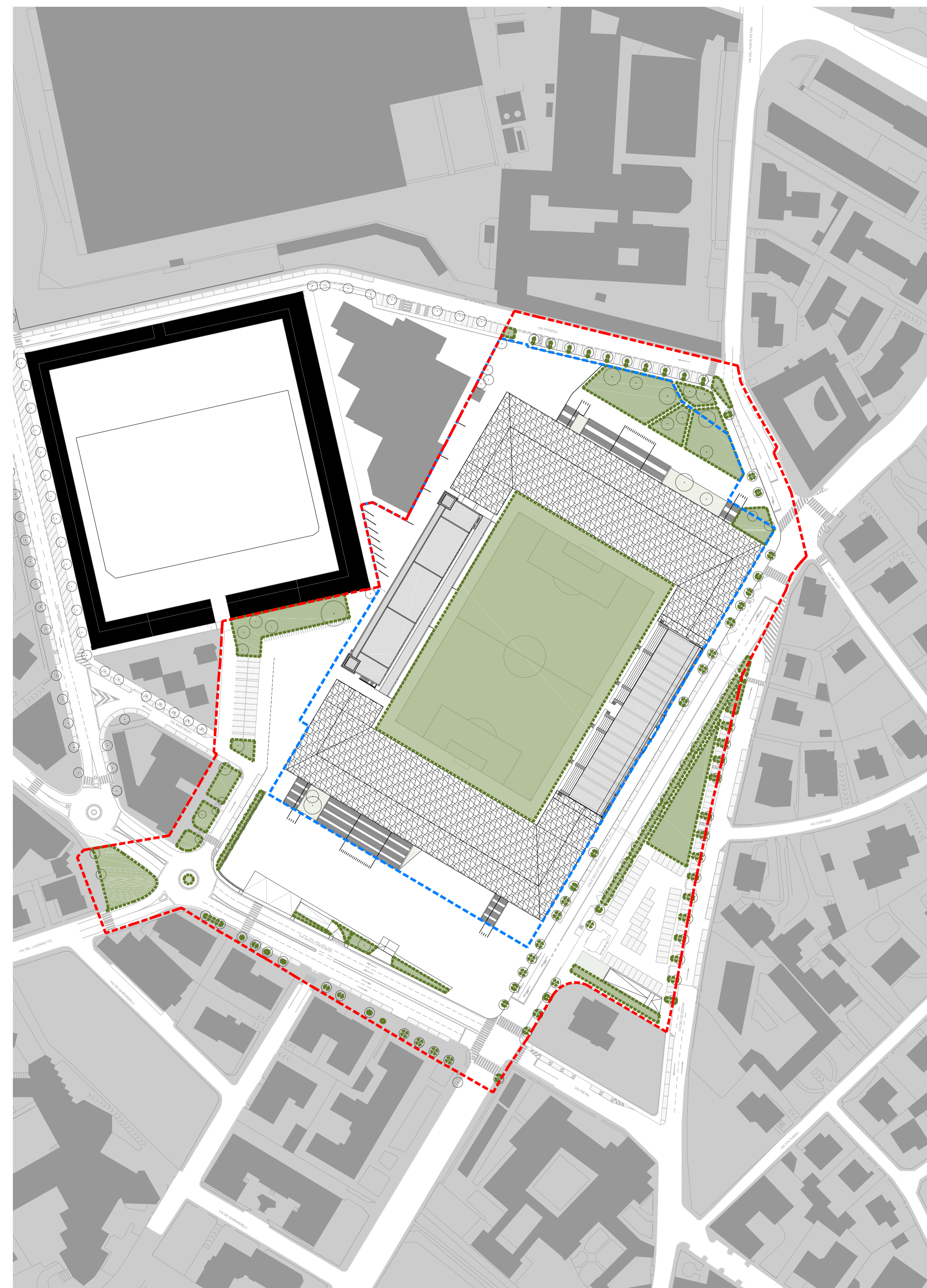
Planimetria di Progetto - Calcolo superficie drenante
