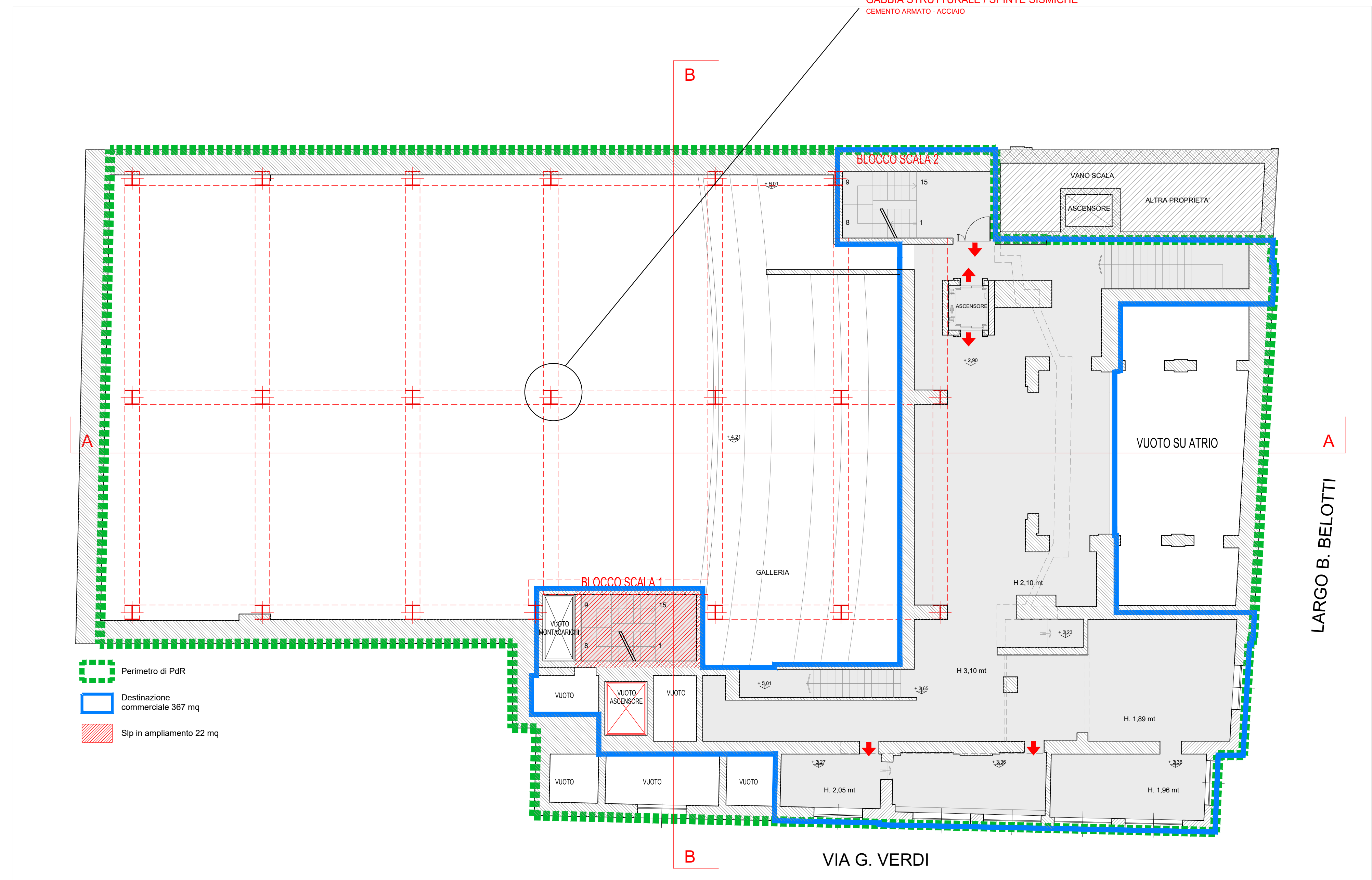
PLANIMETRIA PIANO AMMEZZATO
