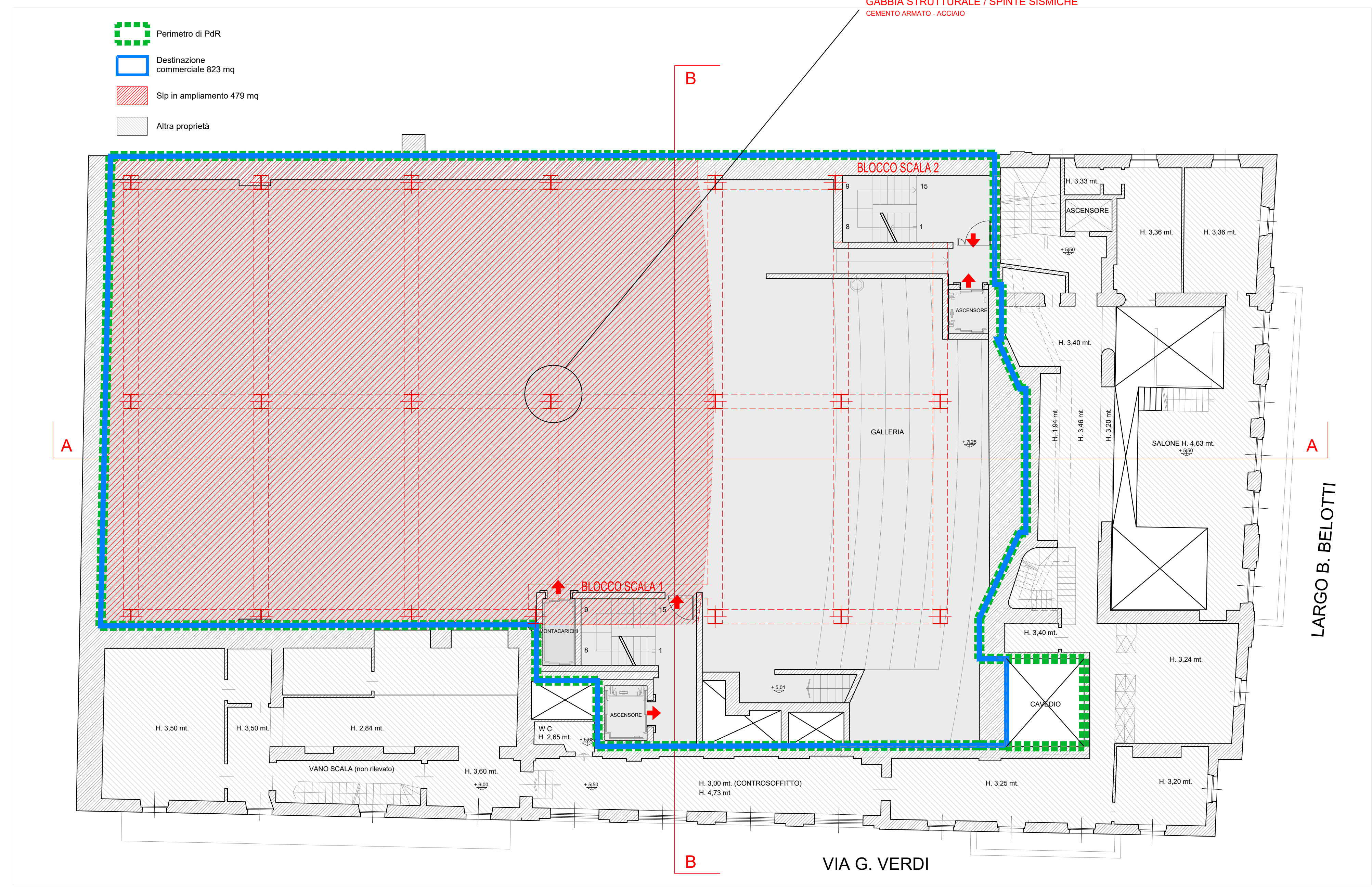
PLANIMETRIA PIANO PRIMO
