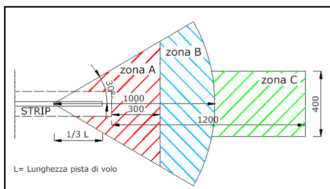
Figura 1 - Zone di tutela per piste di volo di codice 1 e 2 (estratto dal Regolamento ENAC)
